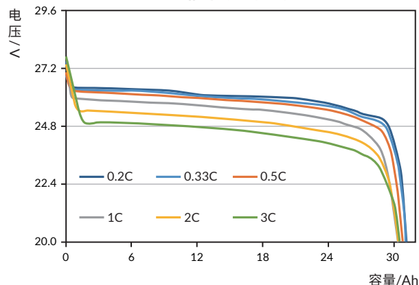
倍率放电曲线
